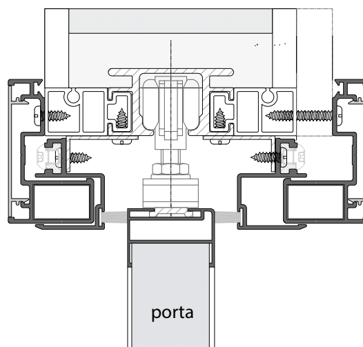
Telaio porta scorrevole profilo linear
