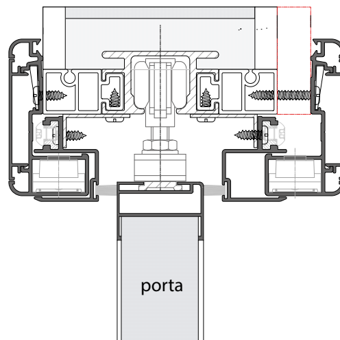
Telaio porta scorrevole profilo standard
