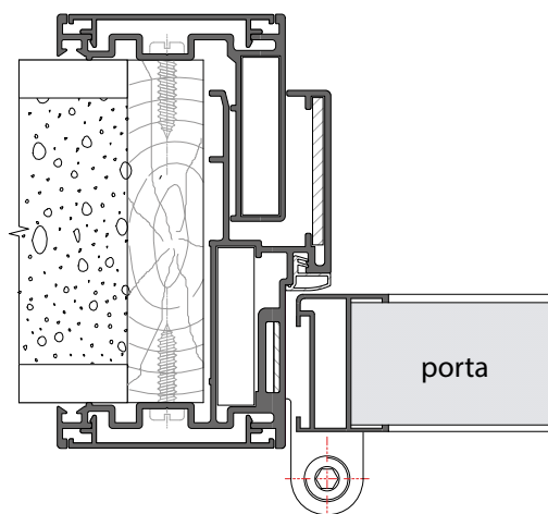
Telaio porta battente profilo linear
