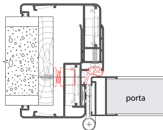
Telaio porta battente profilo standard
